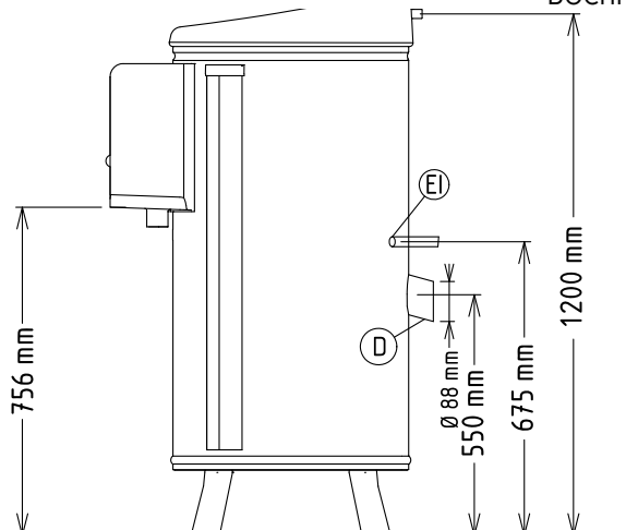
Boční
